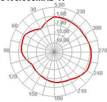
5490.000MHz H
