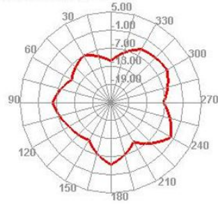
5150.000MHz H
