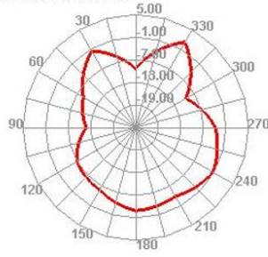
2450.000MHz H
