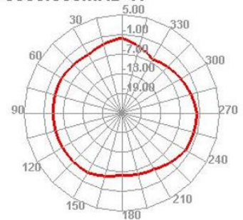
5850.000MHz H
