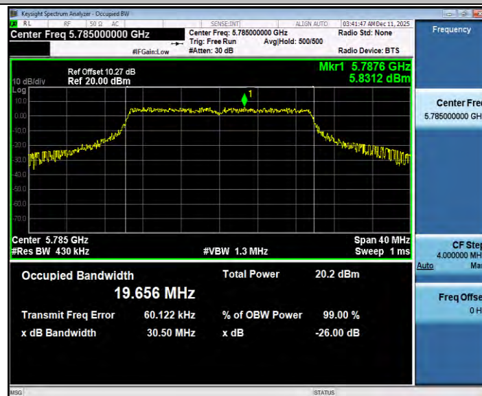
11AX20ISO_Ant1_5785
