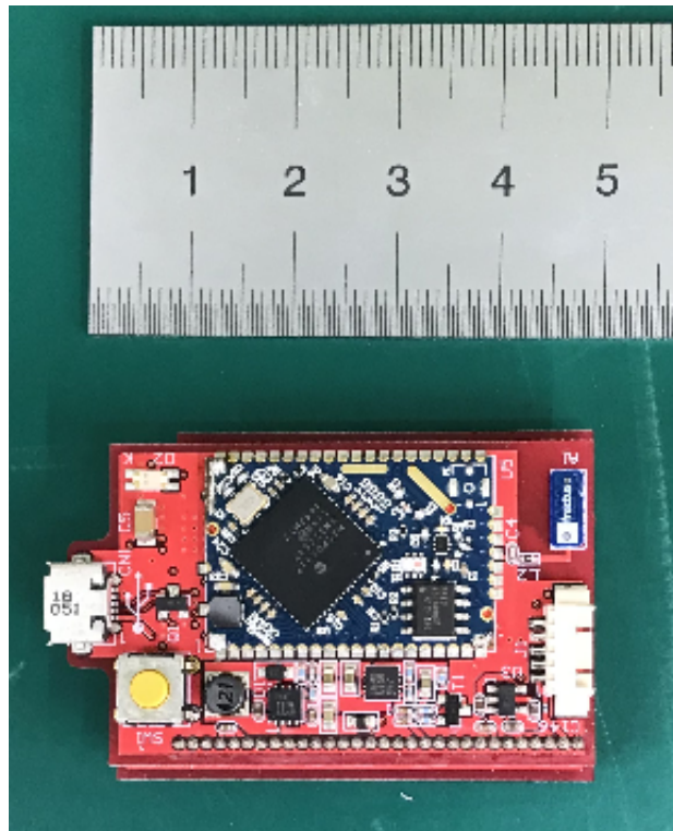
Wi-Fi Module_1
