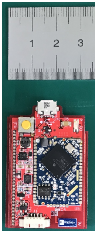
Wi-Fi Module_2
