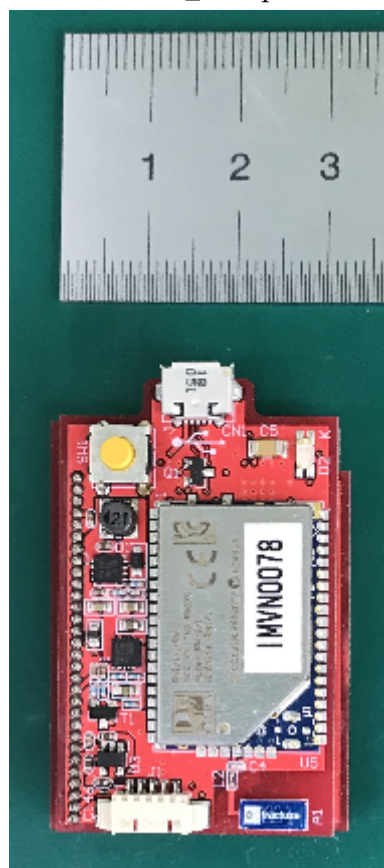
PCB_2 : Top
