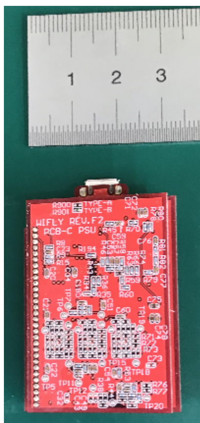
PCB_4: Bottom
