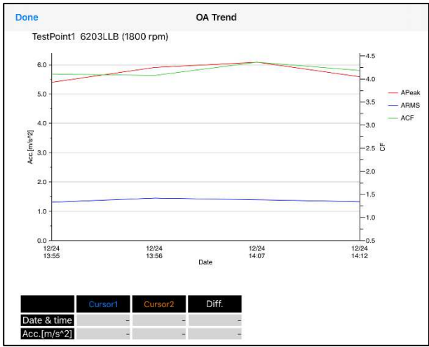
Figure 4.39 OA Trend
