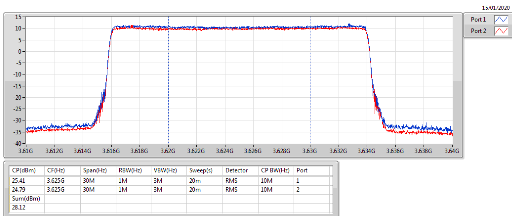
Band 48_LTE_20MHz_Nss1,QPSK_2TX 3625MHz_QPSK_RB 100,#RB 0
