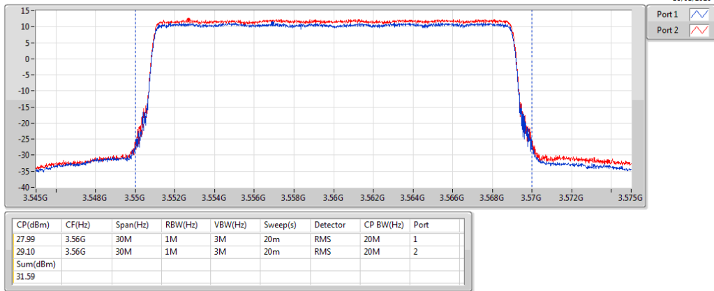
Band 48_LTE_20MHz_Nss1,QPSK_2TX 3560MHz_QPSK_RB 100,#RB 0
