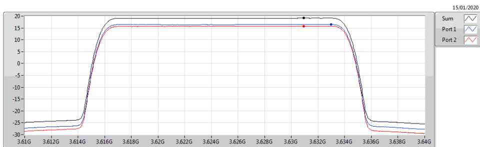
Band 48_LTE_20MHz_Nss1,QPSK_2TX 3625MHz_QPSK_RB 100,#RB 0
