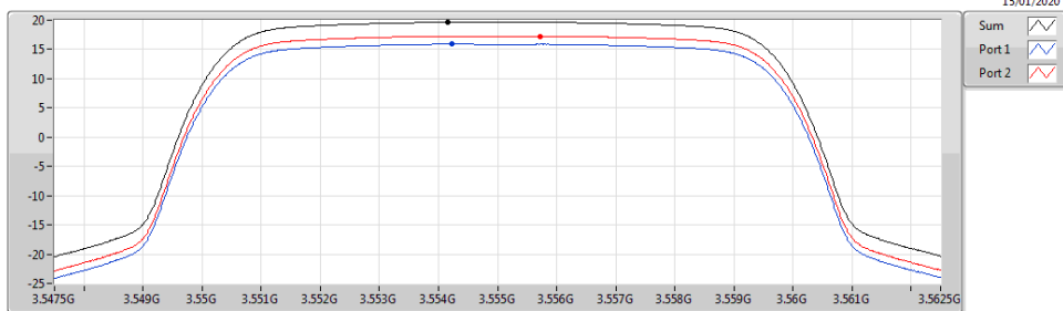
Band 48_LTE_10MHz_Nss1,QPSK_2TX 3555MHz_QPSK_RB 50,#RB 0
