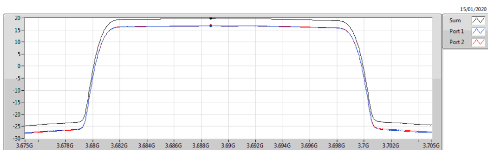
Band 48_LTE_20MHz_Nss1,QPSK_2TX 3690MHz_QPSK_RB 100,#RB 0
