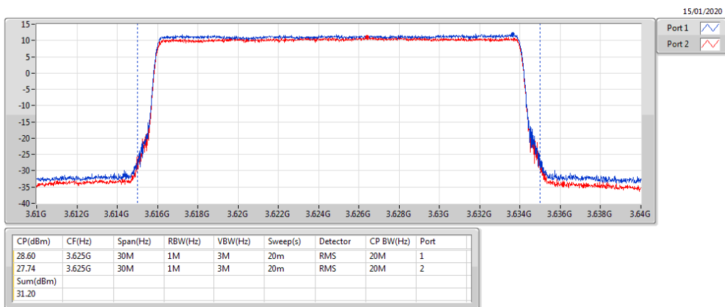
Band 48_LTE_20MHz_Nss1,QPSK_2TX 3625MHz_QPSK_RB 100,#RB 0
