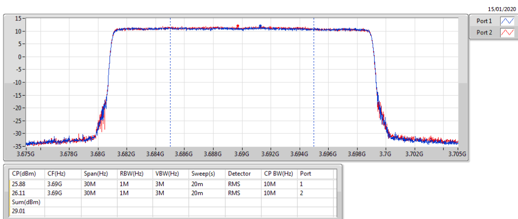
Band 48_LTE_20MHz_Nss1,QPSK_2TX 3690MHz_QPSK_RB 100,#RB 0
