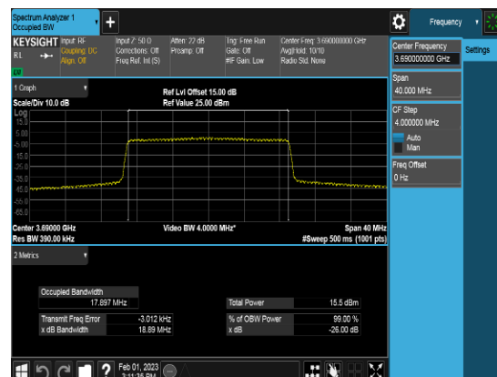
SCC_20M_3690MHz_QPSK_FULLLRB_OBW
