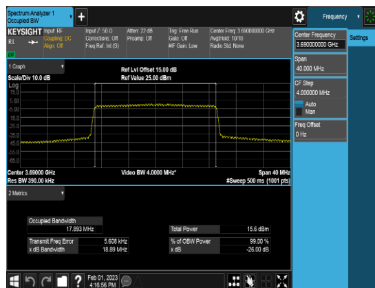
SCC_20M_3690MHz_QPSK_FULLLRB_OBW
