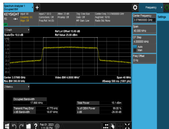
SCC_20M_3579.8MHz_QPSK_FULLLRB_OBW
