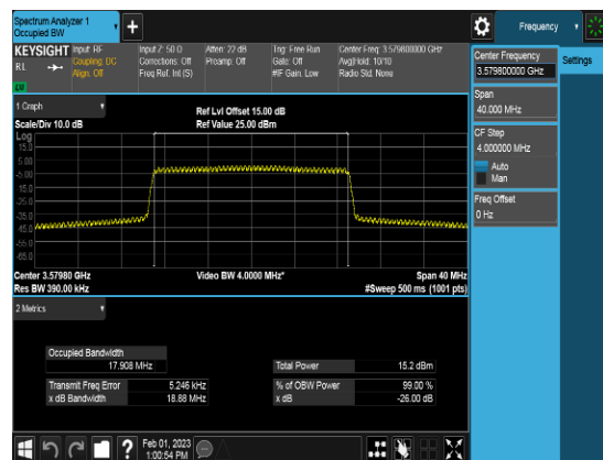
SCC_20M_3579.8MHz_QPSK_FULLLRB_OBW
