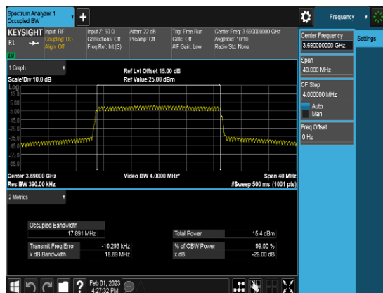
SCC_20M_3690MHz_QPSK_FULLLRB_OBW
