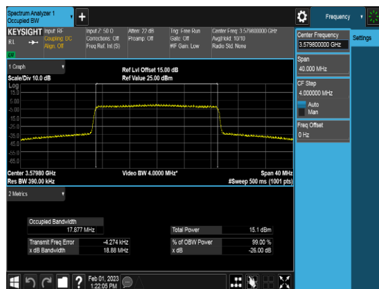
SCC_20M_3579.8MHz_Q64_FULLLRB_OBW
