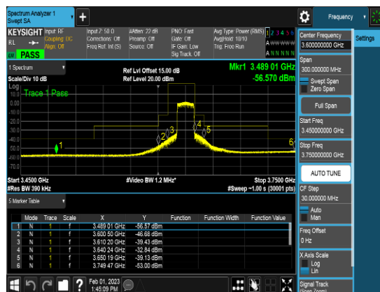
SCC_20M_3630MHz_Q16_FULLLRB_CSEpart96
