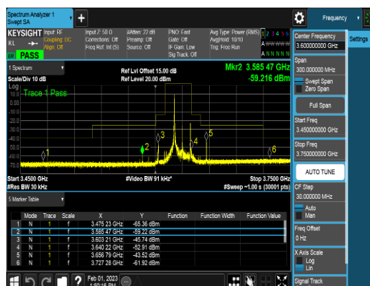
SCC_20M_3630MHz_Q16_1RB_CSEpart96
