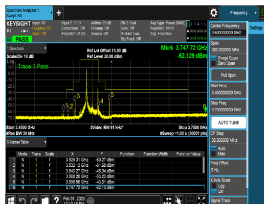
SCC_20M_3569.9MHz_Q16_1RB_CSEpart96
