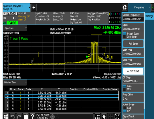
PCC_20M_3680.1MHz_Q16_FULLLRB_CSEpart9 6
