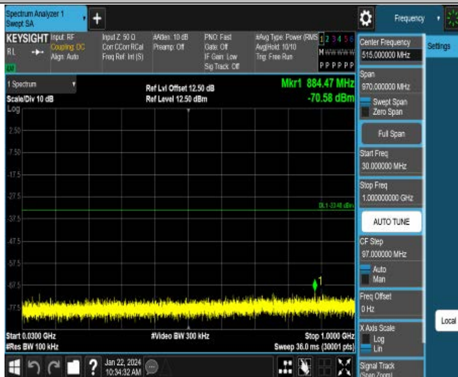
11N20MIMO_Ant1_2412_30~1000
