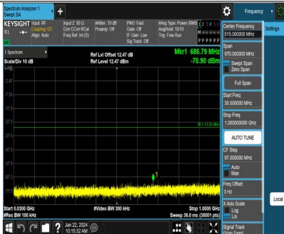
11G-CDD_Ant1_2462_30~1000
