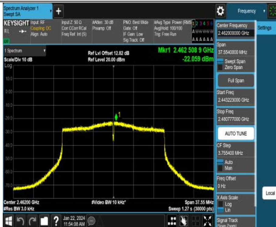
11AX20MIMO_Ant2_2462
