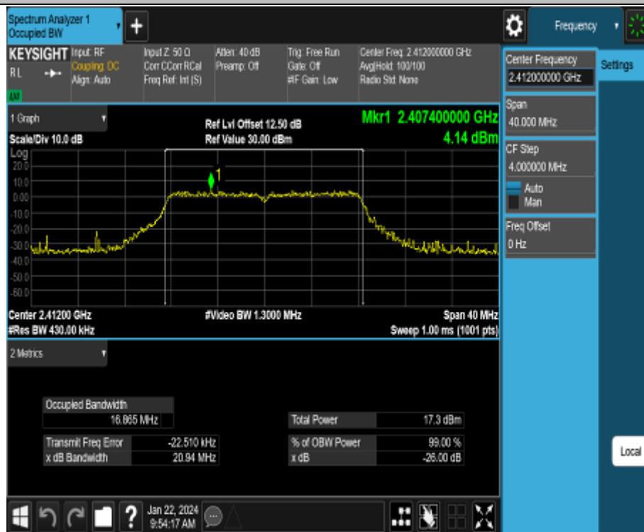
11G-CDD_Ant2_2412
