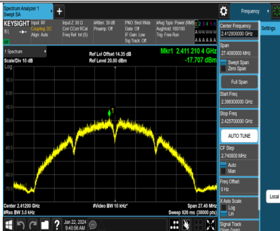
11B-CDD_Ant2_2412
