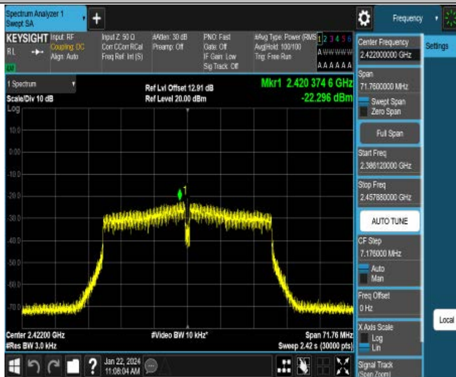
11N40MIMO_Ant2_2422
