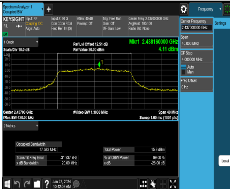
11N20MIMO_Ant2_2437
