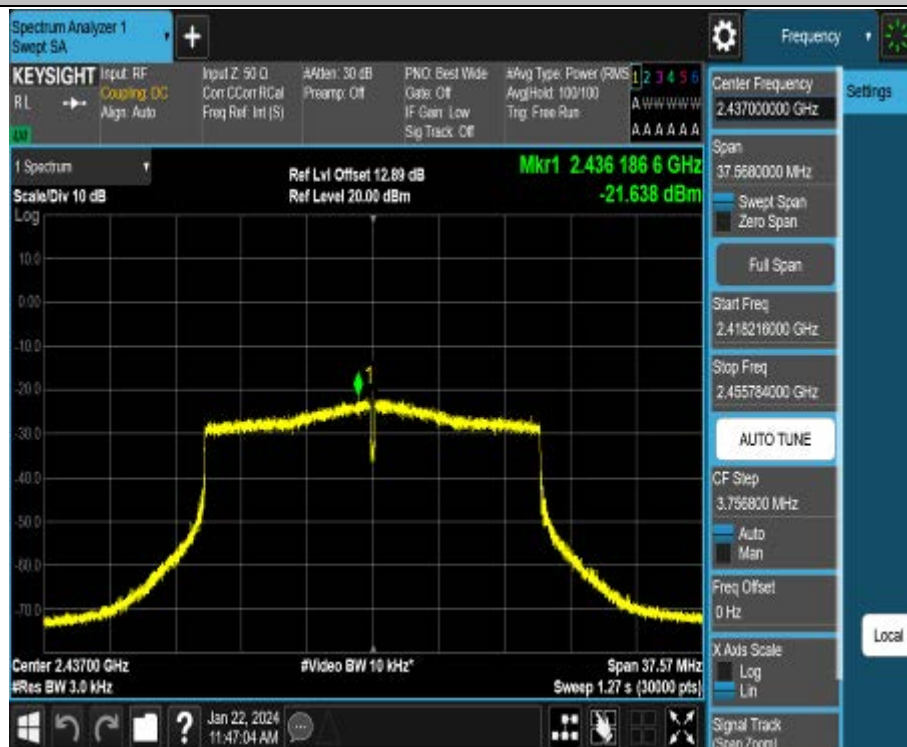
11AX20MIMO_Ant2_2437
