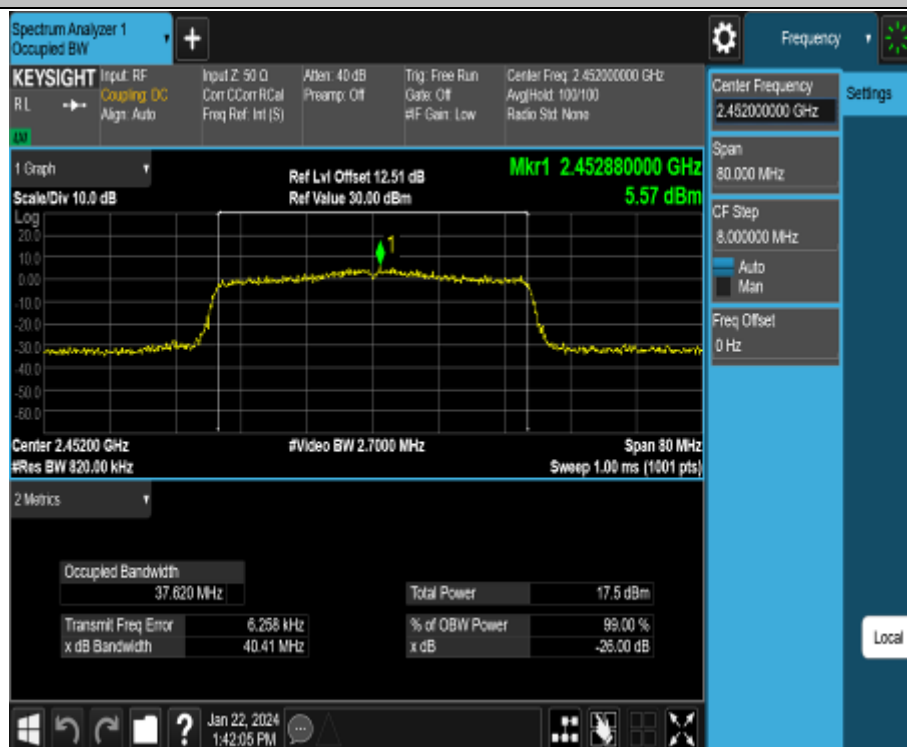
11AX40MIMO_Ant2_2452
