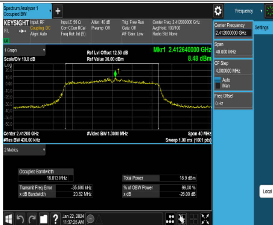
11AX20MIMO_Ant2_2412
