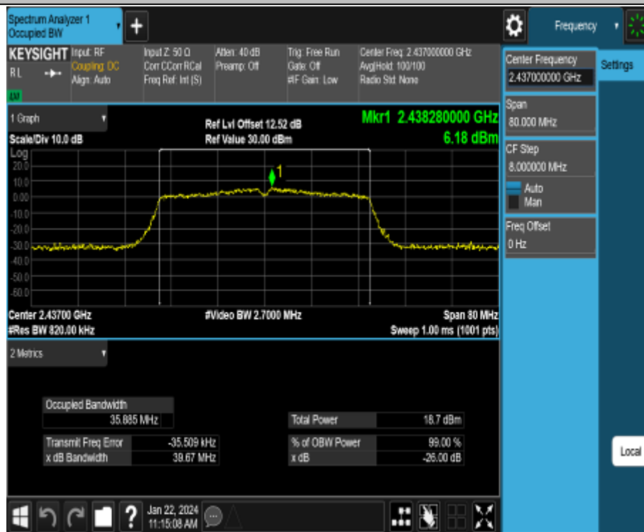
11N40MIMO_Ant2_2437
