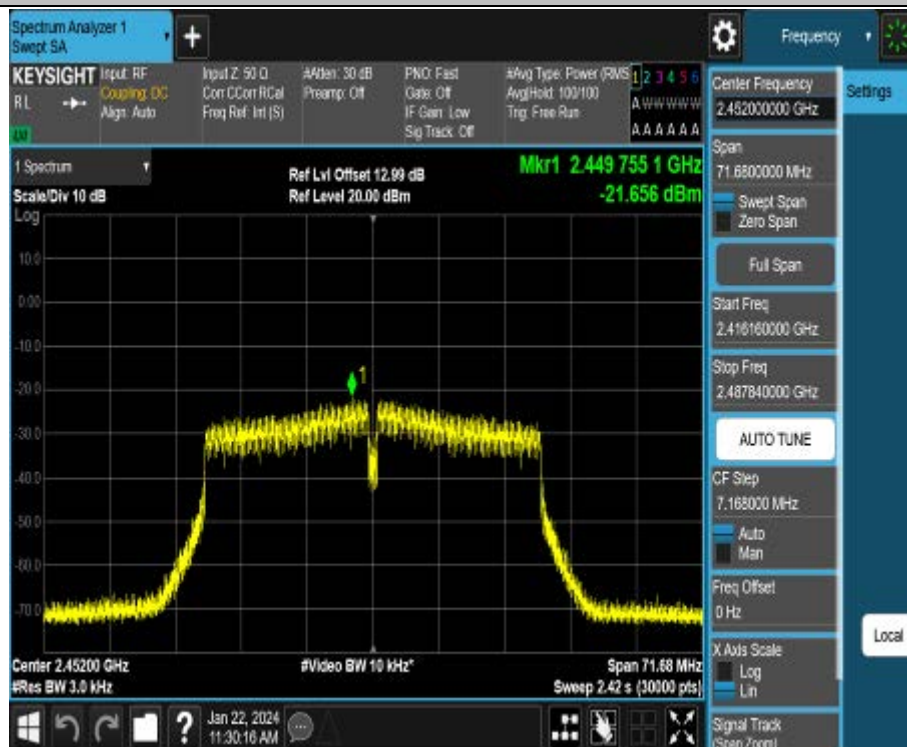
11N40MIMO_Ant2_2452
