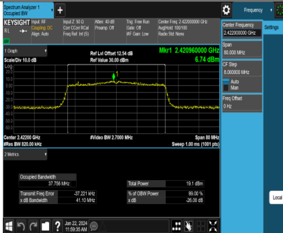
11AX40MIMO_Ant2_2422
