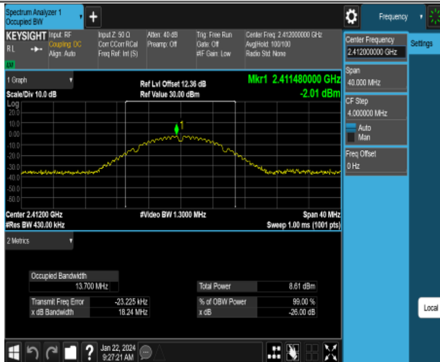
11B-CDD_Ant2_2412
