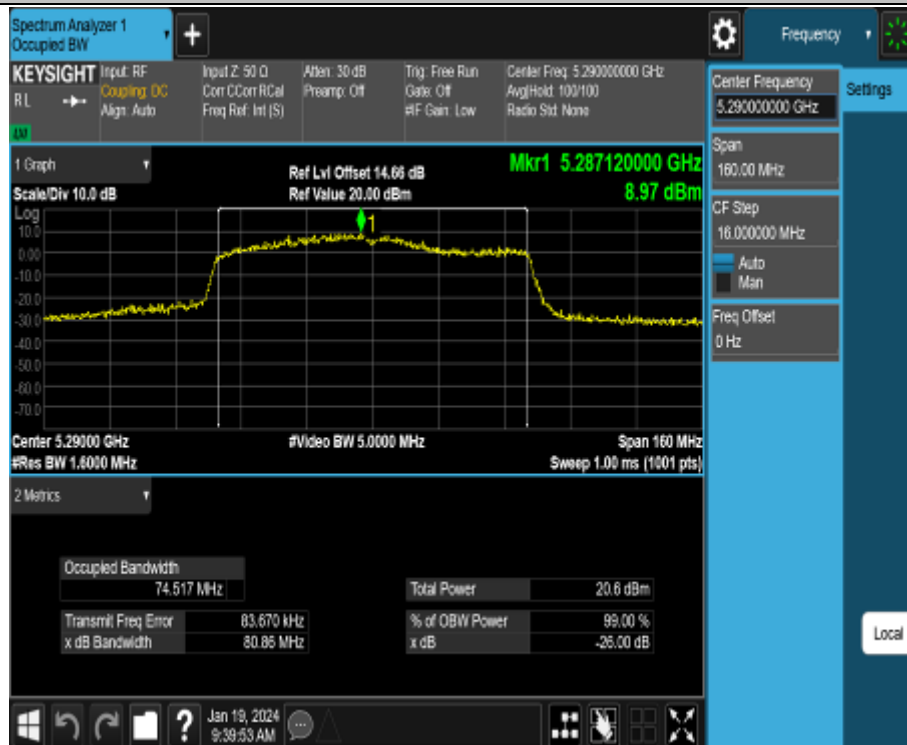
11AC80MIMO_Ant2_5290
