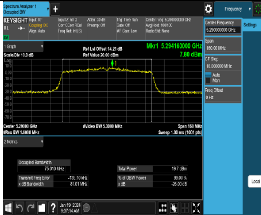
11AC80MIMO_Ant2_5290
