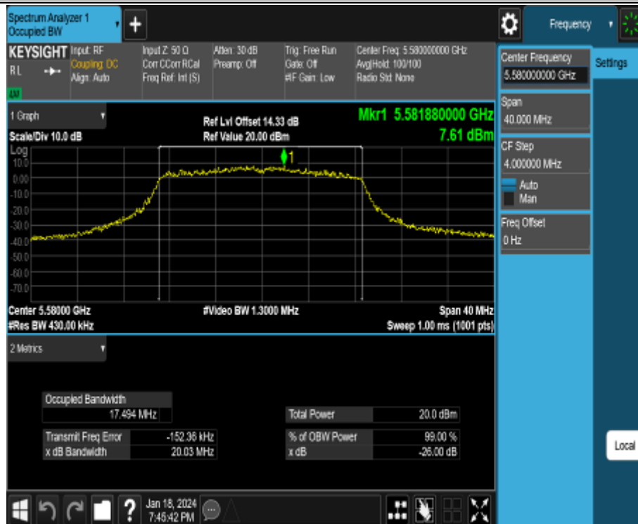
11AC20MIMO_Ant2_5580
