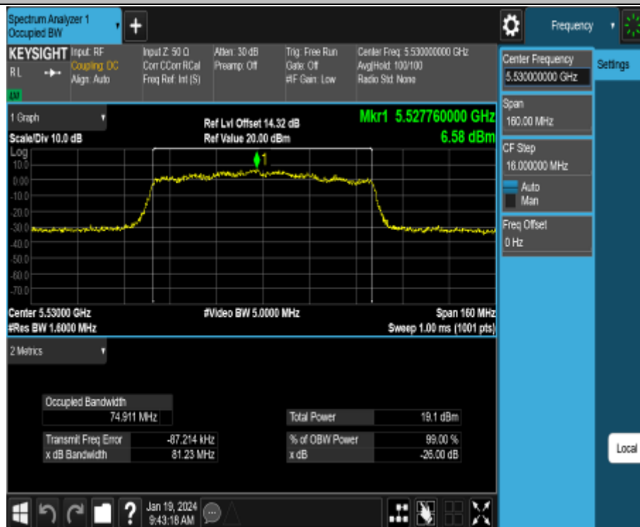
11AC80MIMO_Ant2_5530
