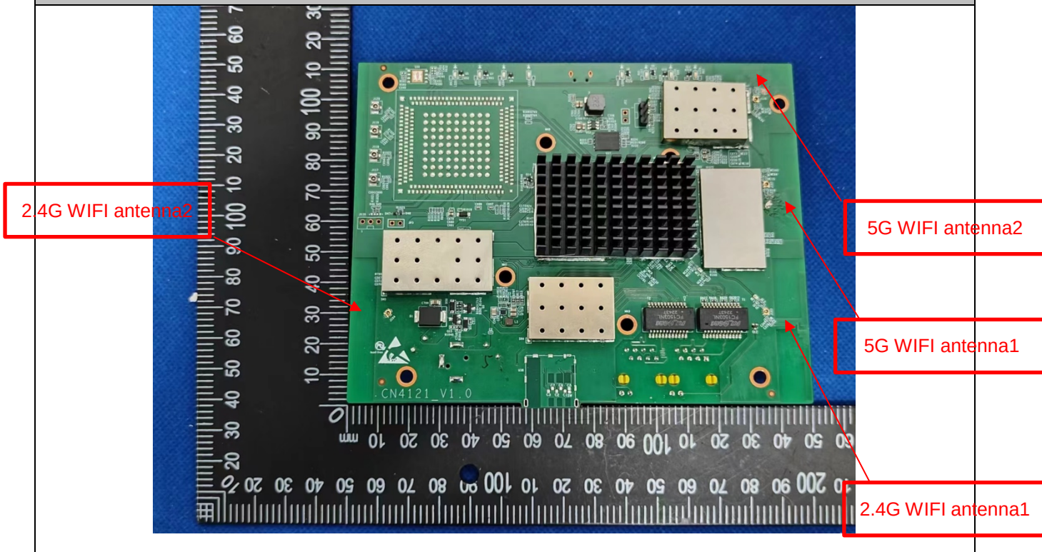
EUT Photo
