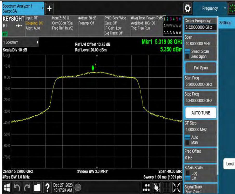
11AX20MIMO_Ant2_5320
