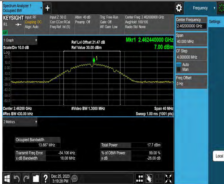
11B-CDD_Ant2_2462
