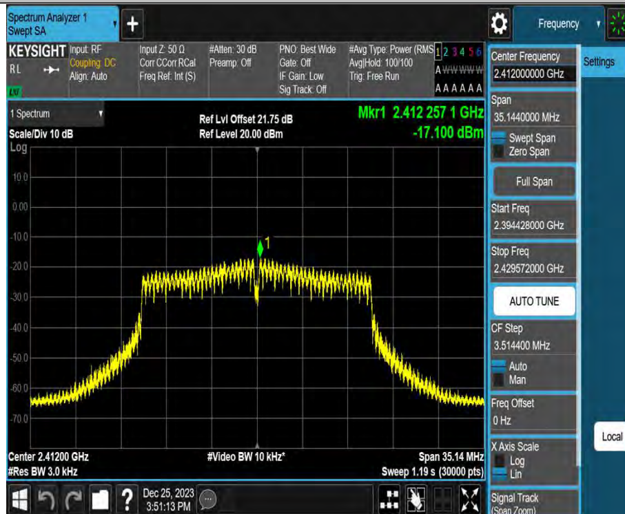
11N20MIMO_Ant2_2412
