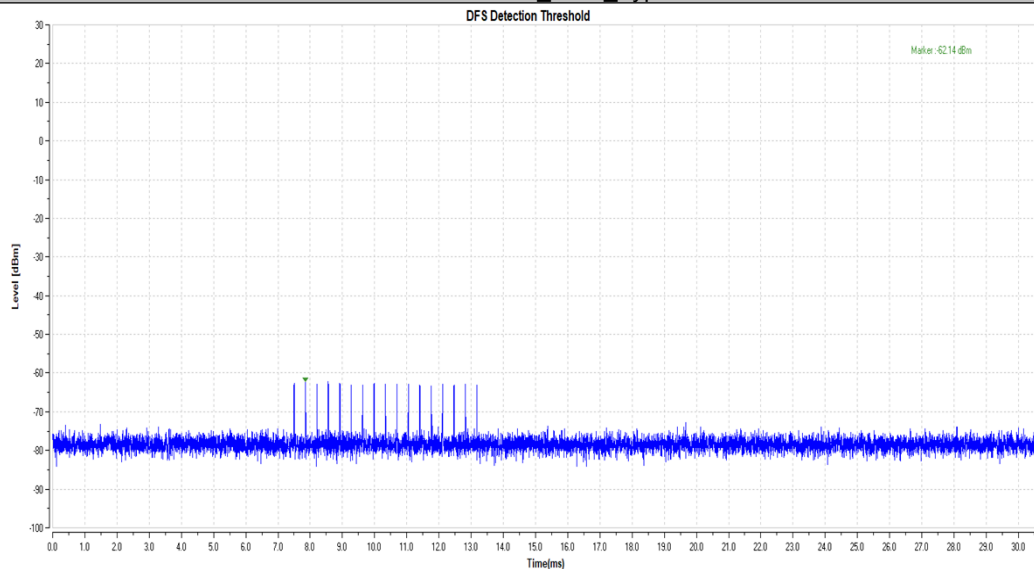
11AX160MIMO_5250_Type4
