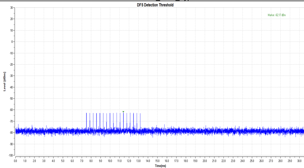
11AX20MIMO_5580_Type4
