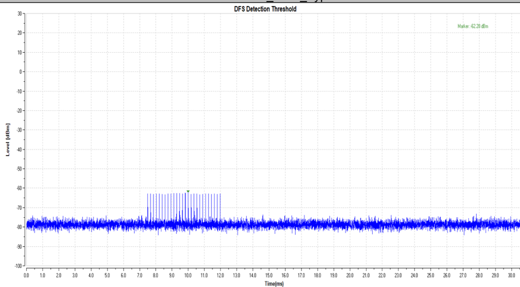
11AX20MIMO_5580_Type2
