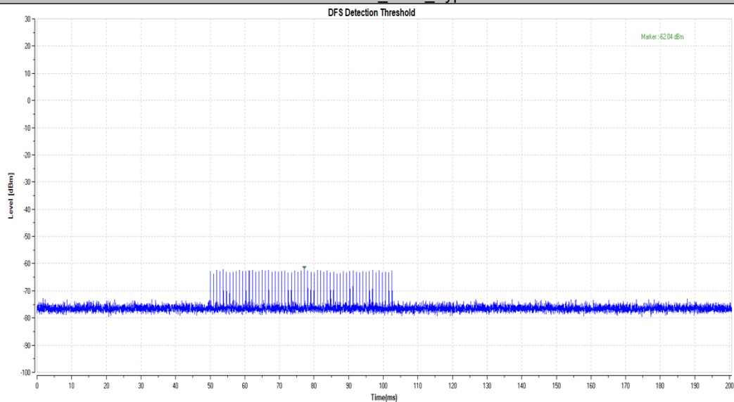
11AX160MIMO_5250_Type1
