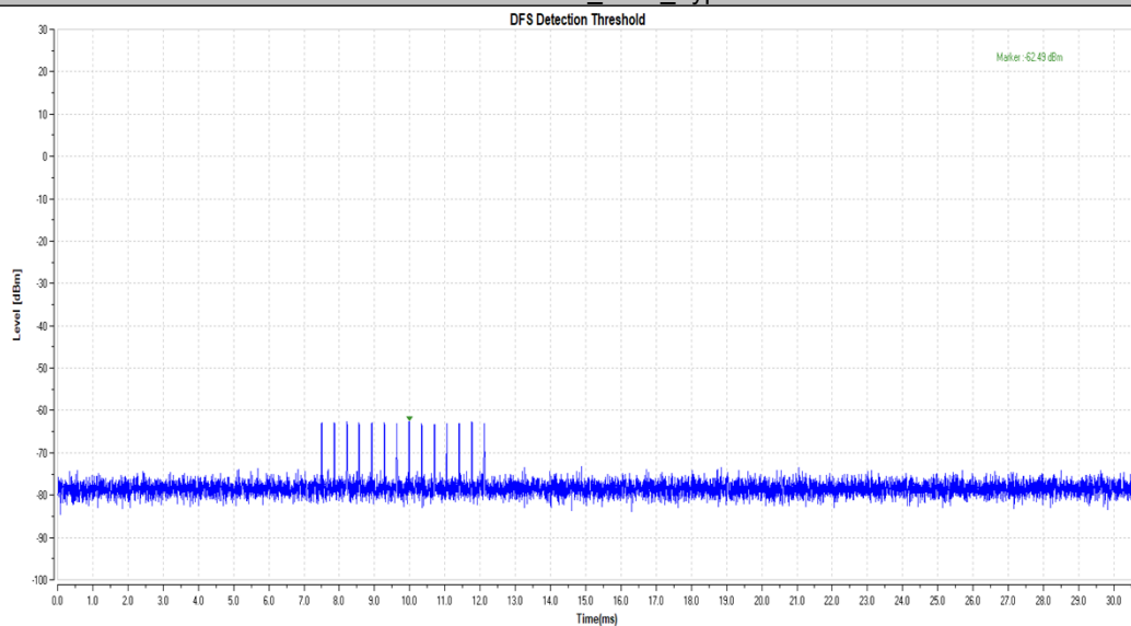
11AX160MIMO_5250_Type4
