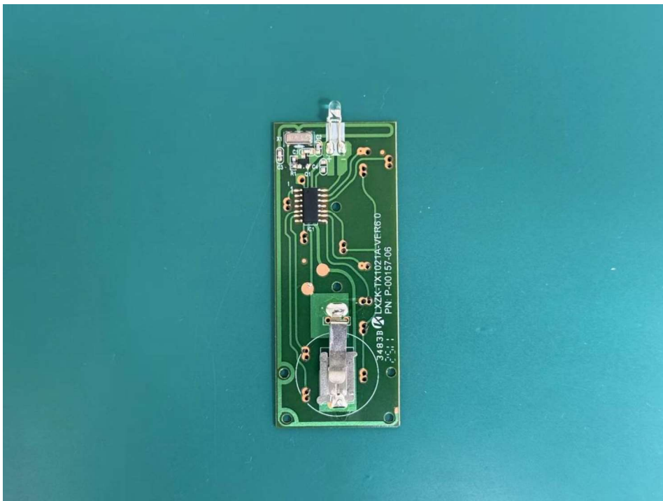
Internal: Bottom
