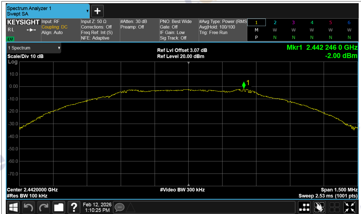
Tx. Spurious NVNT BLE 1M 2442MHz Ant1 Emission
