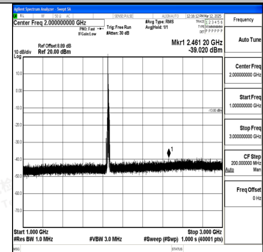
Band2_10MHz_QPSK_18650_1RB#0_1000~300 0_1000~3000
