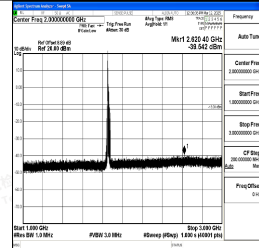
Band2_15MHz_QPSK_18675_1RB#0_1000~300 0_1000~3000
