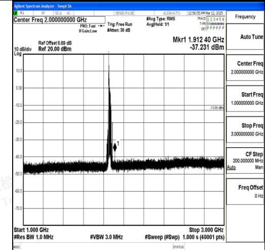
Band2_20MHz_QPSK_18700_1RB#0_1000~300 0_1000~3000
