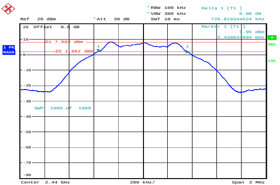
Middle 0.726MHz
