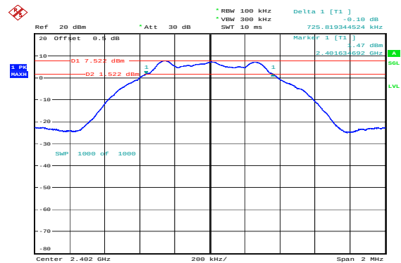
Low 0.726MHz
