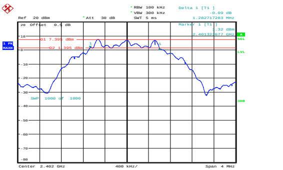
Low 1.283MHz
