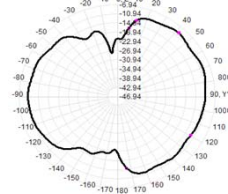
2490.0MHz Total(E2-YZ), Max=-10.71dB
