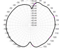
2500.0MHz Total(E2-YZ), Max=-10.48dB
