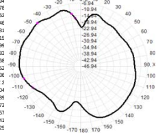
2490.0MHz Total(E1-XZ), Max=-10.69dB
