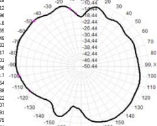
2500.0MHz Total(E1-XZ), Max=-10.43dB
