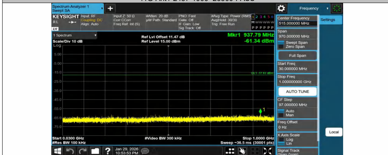
11G-Ant1-2462-30~1000-PASS
