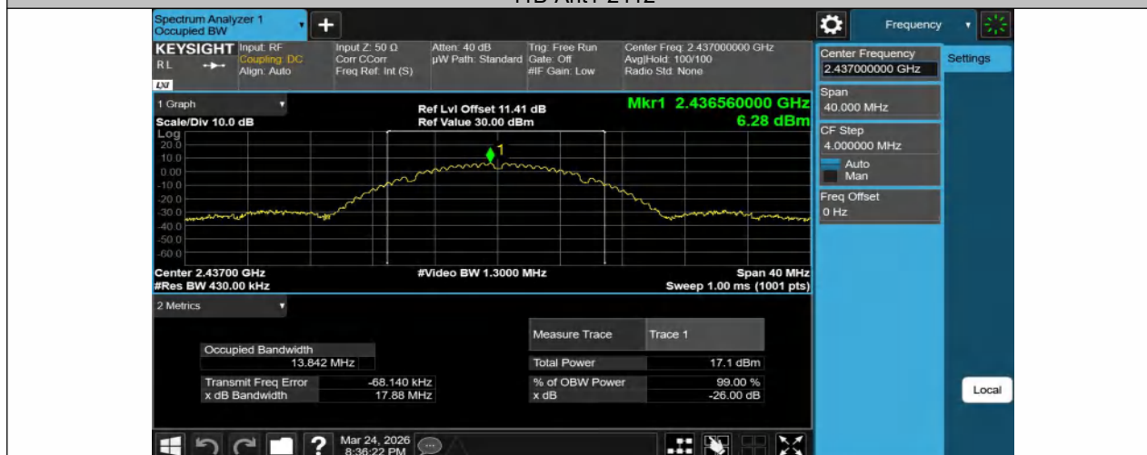
11B-Ant1-2437
