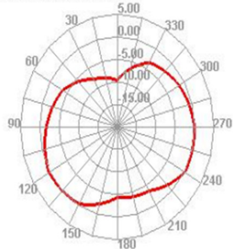
2490.000MHz H
