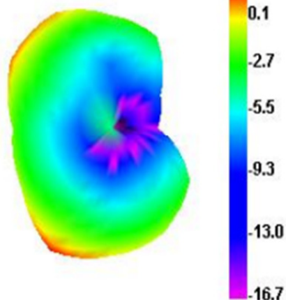
2440.000MHz
