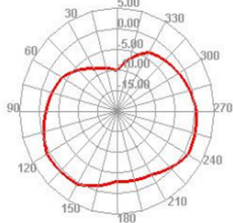
2470.000MHz H
