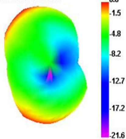
2480.000MHz
