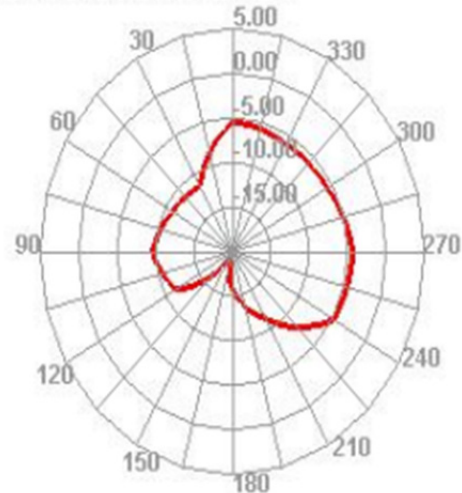
2490.000MHz E1
