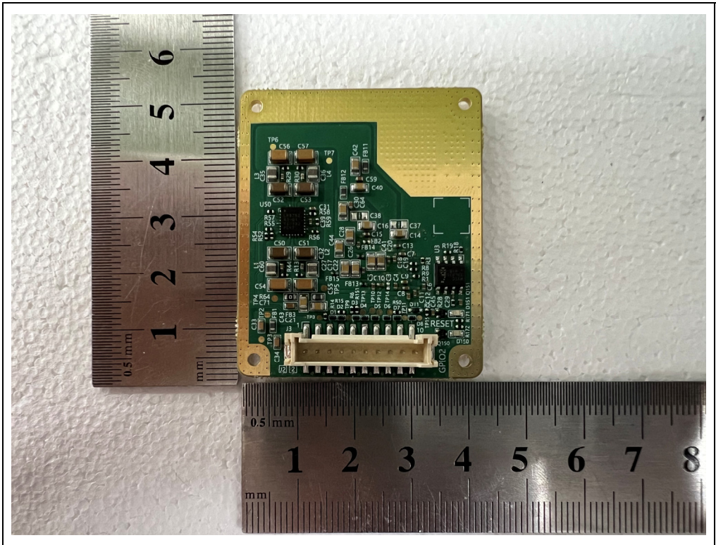
<Antenna>
