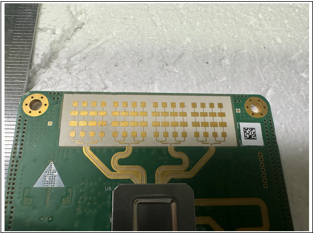
<RX Antenna>
