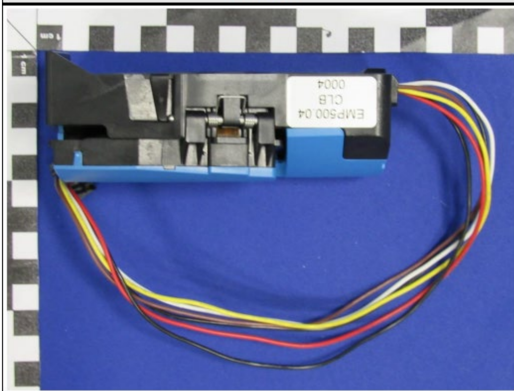
EUT top
