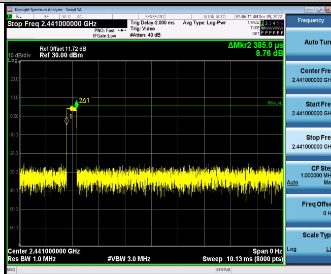
2DH3_Ant1_Hop
