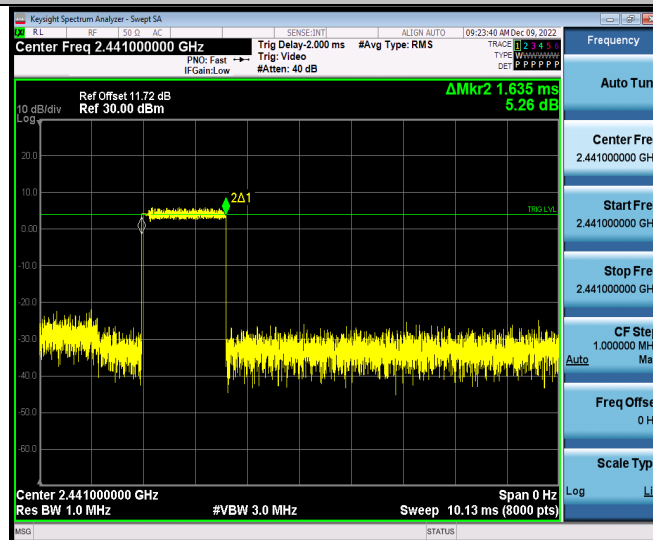
3DH5_Ant1_Hop
