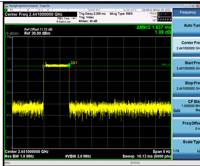
2DH5_Ant1_Hop
