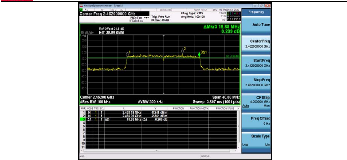
11AX20MIMO_Ant2_2462
