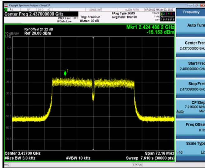
11N40MIMO_Ant2_2437
