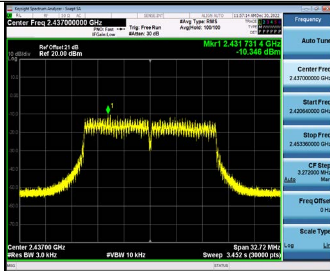
11G-CDD_Ant1_2462
