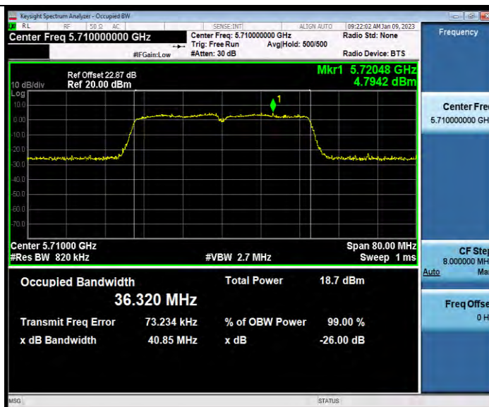
11N40MIMO_Ant2_5710
