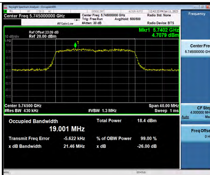
11AX20MIMO_Ant2_5745
