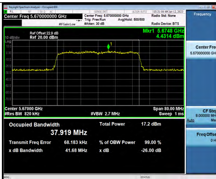
11AX40MIMO_Ant2_5670
