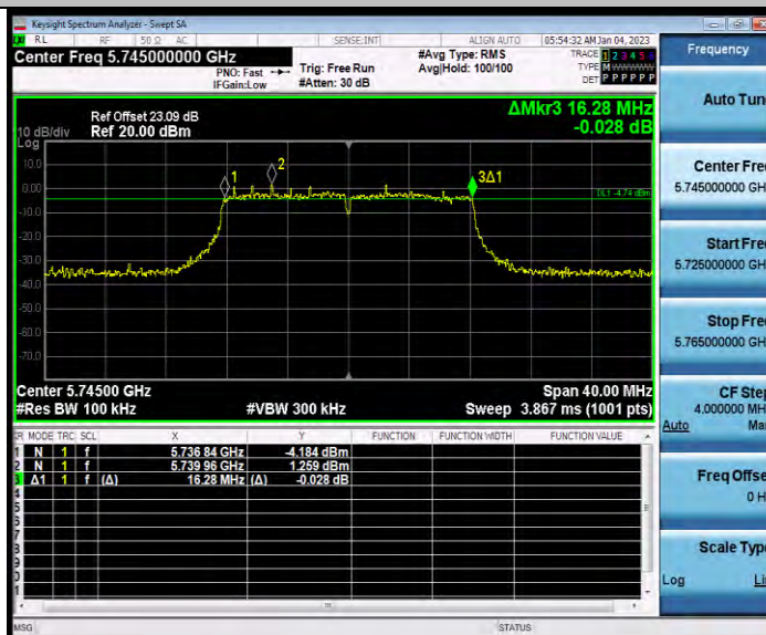
11A-CDD_Ant2_5745
