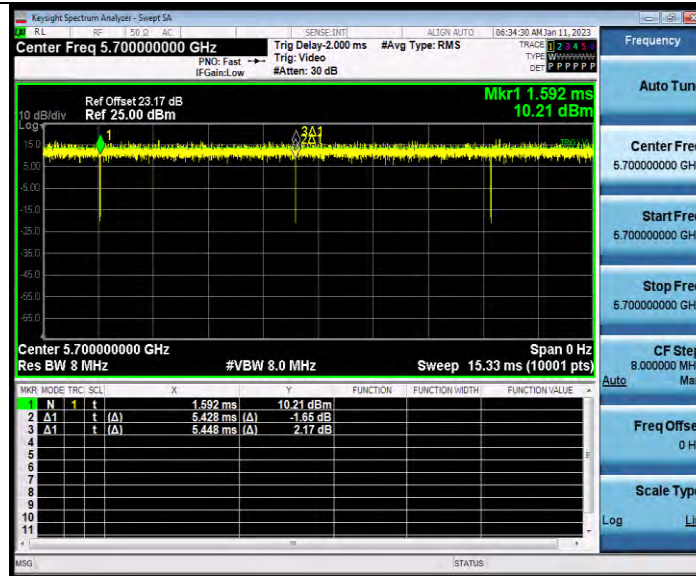
11AC20MIMO_Ant2_5700
