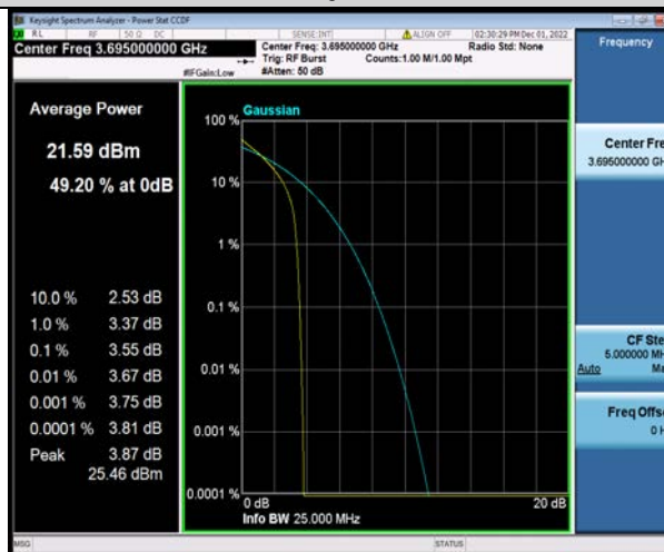
Band48-10MHz-QPSK-56690-50RB#0
