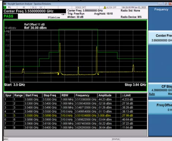
48-48-20MHz-20MHz-QPSK-QPSK-55340-55538-1RB#99-1RB#0
