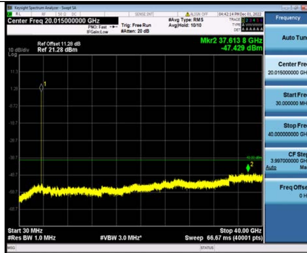
Band48-10MHz-QPSK-55290-1RB#0-Range1:30~40000MHz
