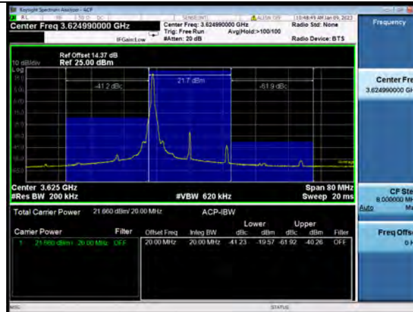
N48-20MHz-QPSK-641666-1RB#50
