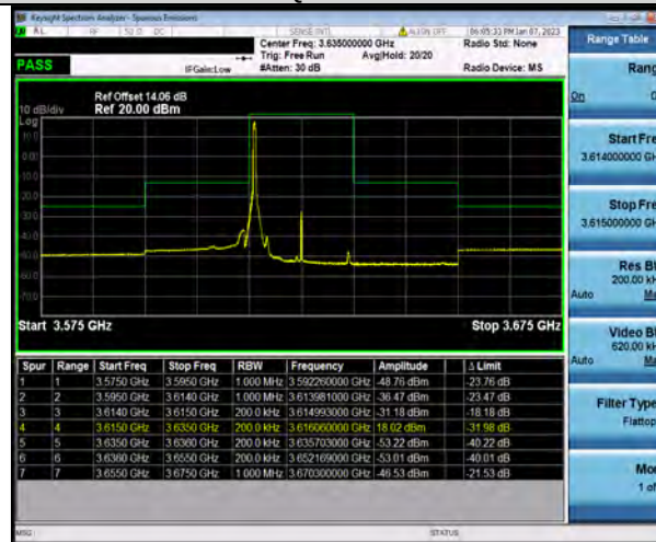
N48-20MHz-QPSK-641666-1RB#50
