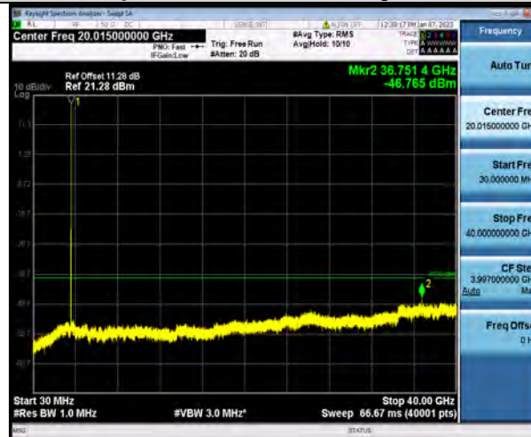
N48-20MHz-QPSK-646000-1RB#0-Range1:30~40000MHz
