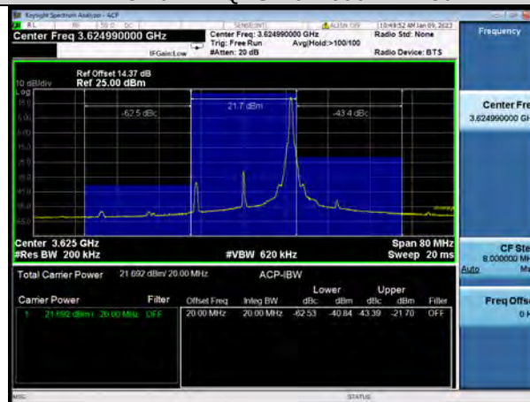
N48-20MHz-QPSK-641666-50RB#0
