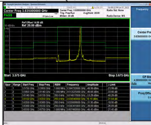
N48-20MHz-QPSK-641666-50RB#0
