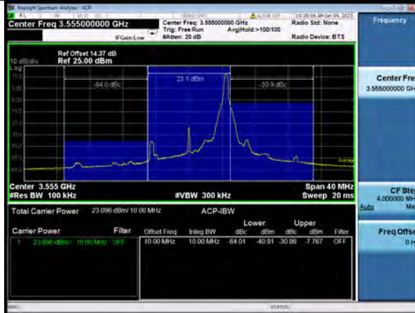
N48-10MHz-QPSK-637000-25RB#0
