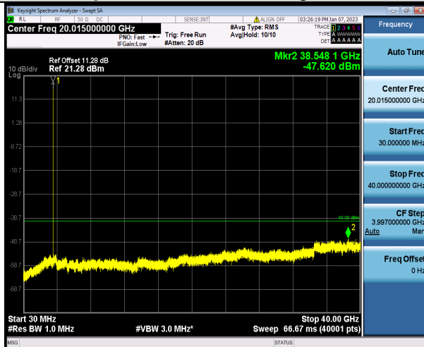
N48-10MHz-QPSK-641666-1RB#0-Range1:30~40000MHz
