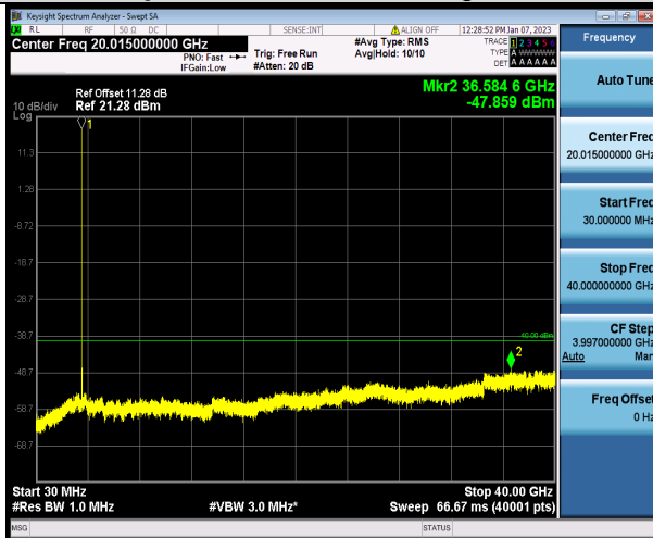
N48-20MHz-QPSK-641666-1RB#0-Range1:30~40000MHz
