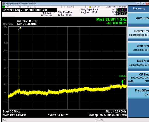
N48-40MHz-QPSK-641666-1RB#0-Range1:30~40000MHz
