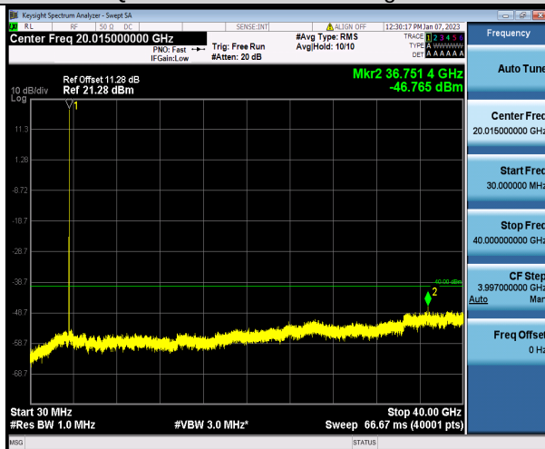
N48-20MHz-QPSK-646000-1RB#0-Range1:30~40000MHz
