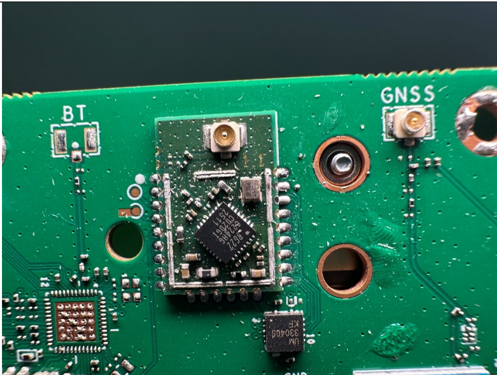
(8) EUT Photo BT Module
