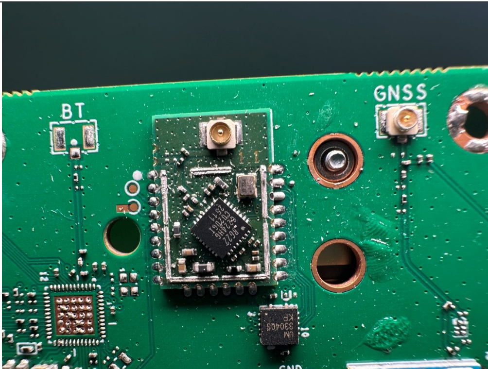
(8) EUT Photo GNSS Module
