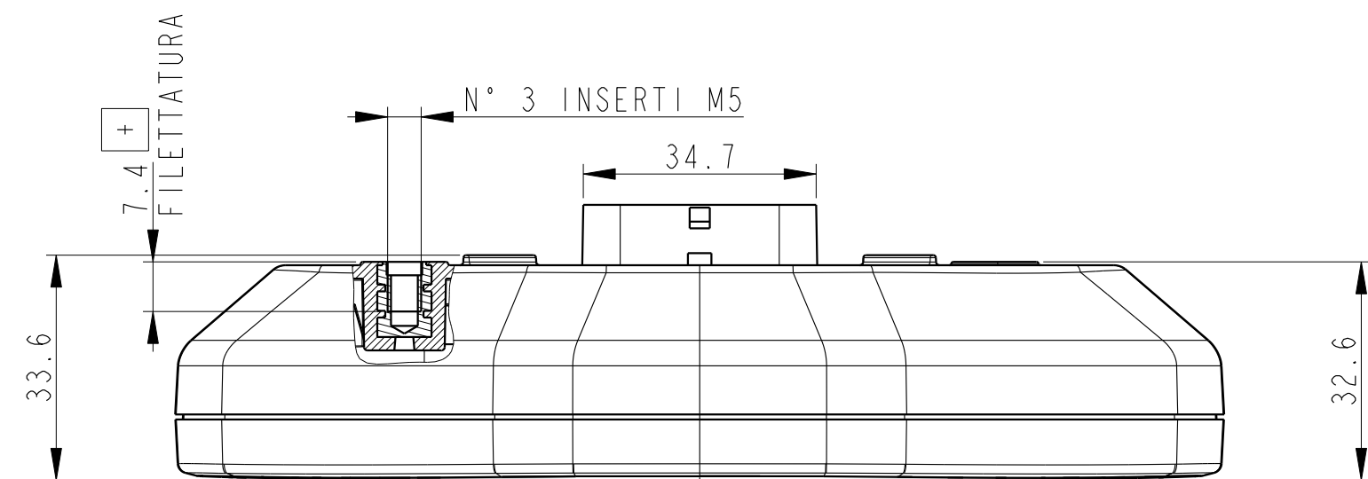
SEZIONE B-B
