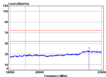
Dongle 2.4G SRD_TX_CH_H_Horizontal
