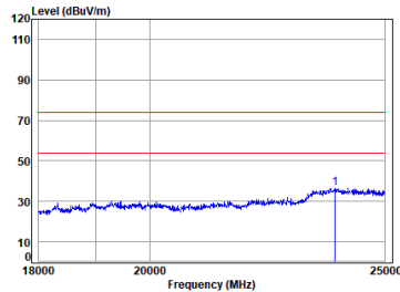
Dongle 2.4G SRD_TX_CH_L_Horizontal
