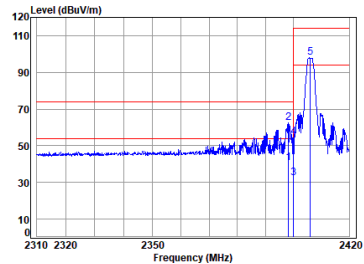
Dongle 2.4G SRD_TX_CH_L_Vertical
