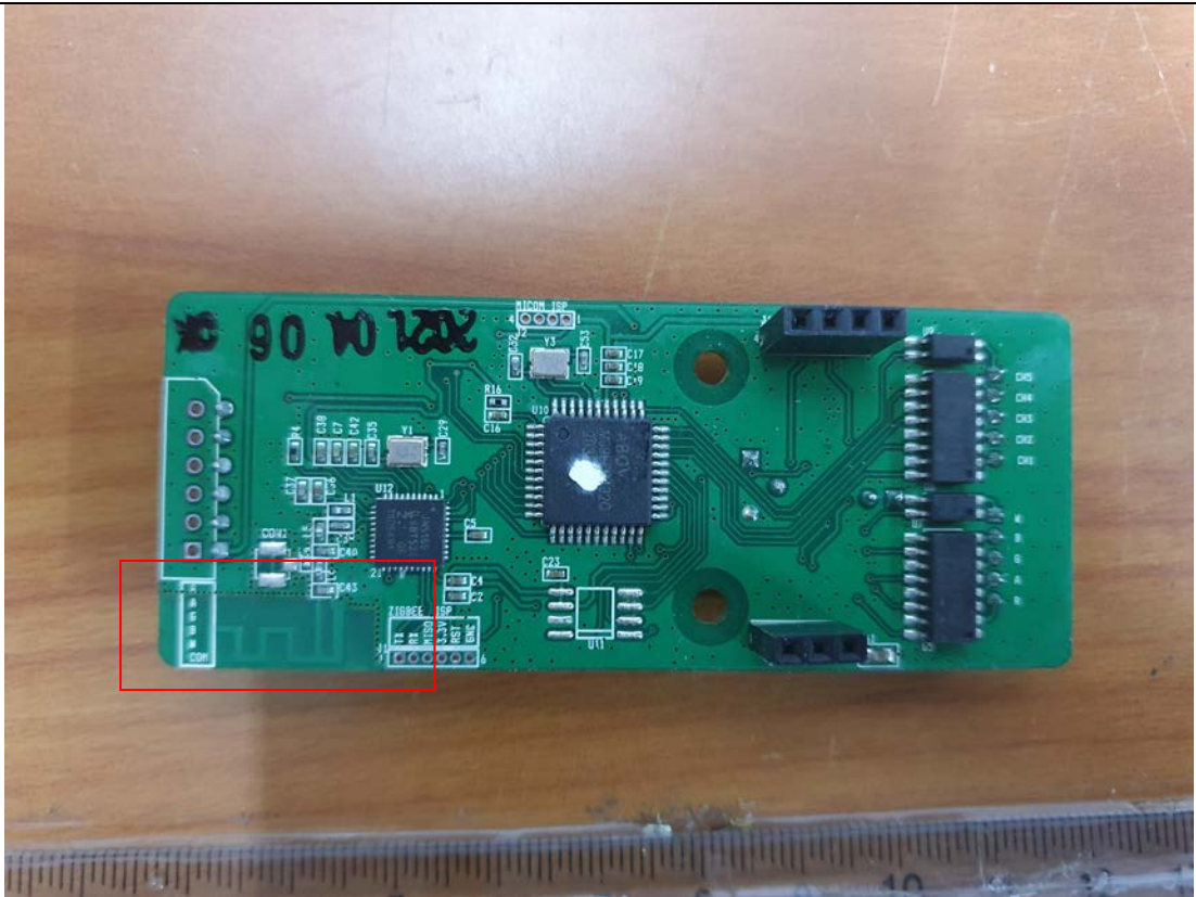
ANTENNA(2.4 GHz)
