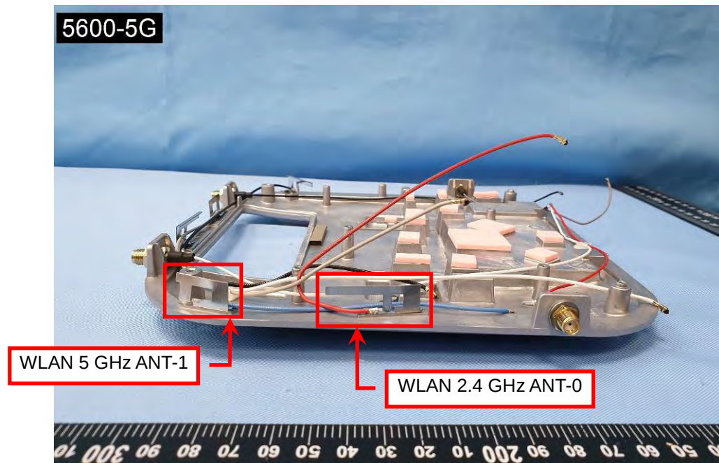
EUT Photo (20)
