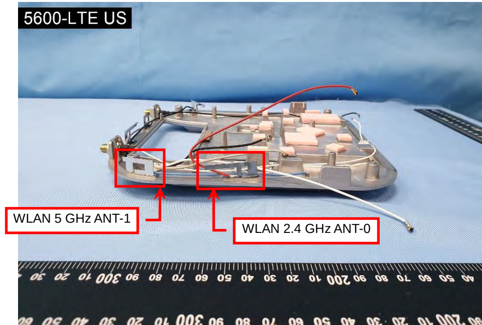
EUT Photo (44)
