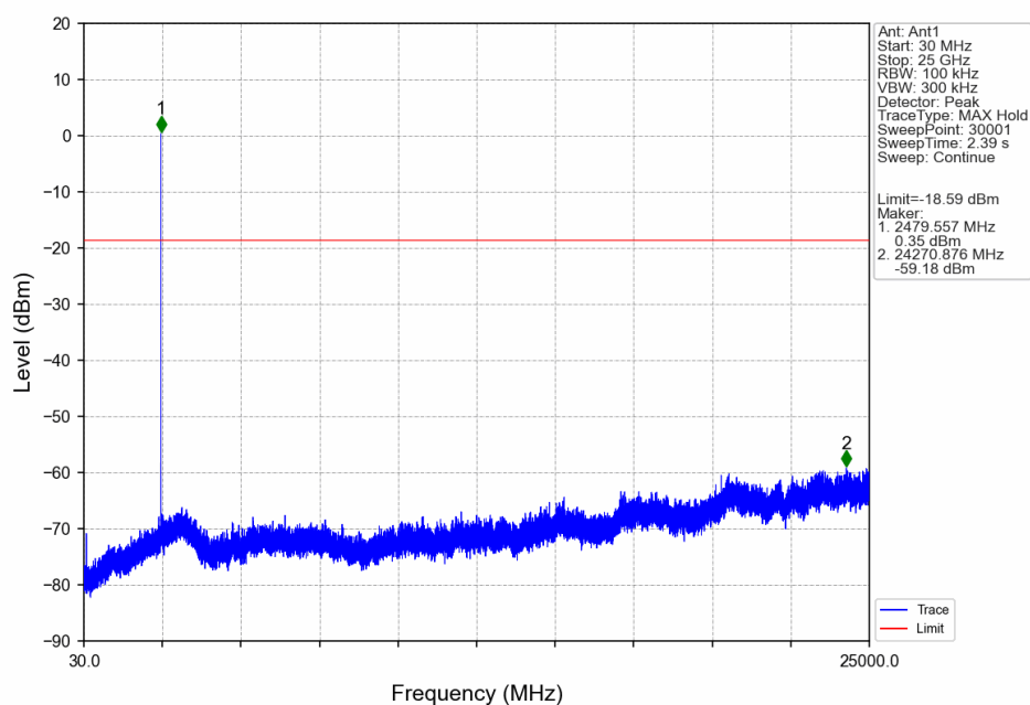
GFSK DH5 HCH 2480MHz Ant1 NTN
