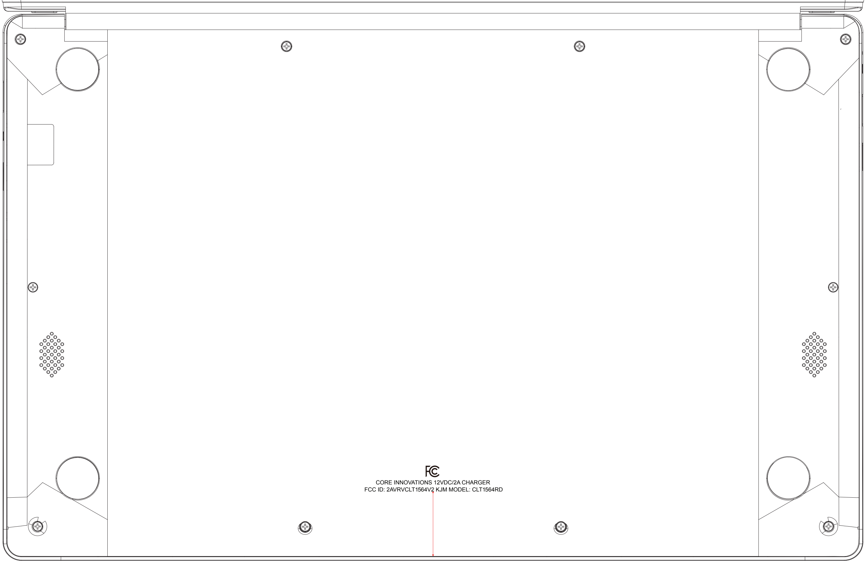
丝印尺寸：54.5x11.16mm 左右居中 丝印颜色：白色
