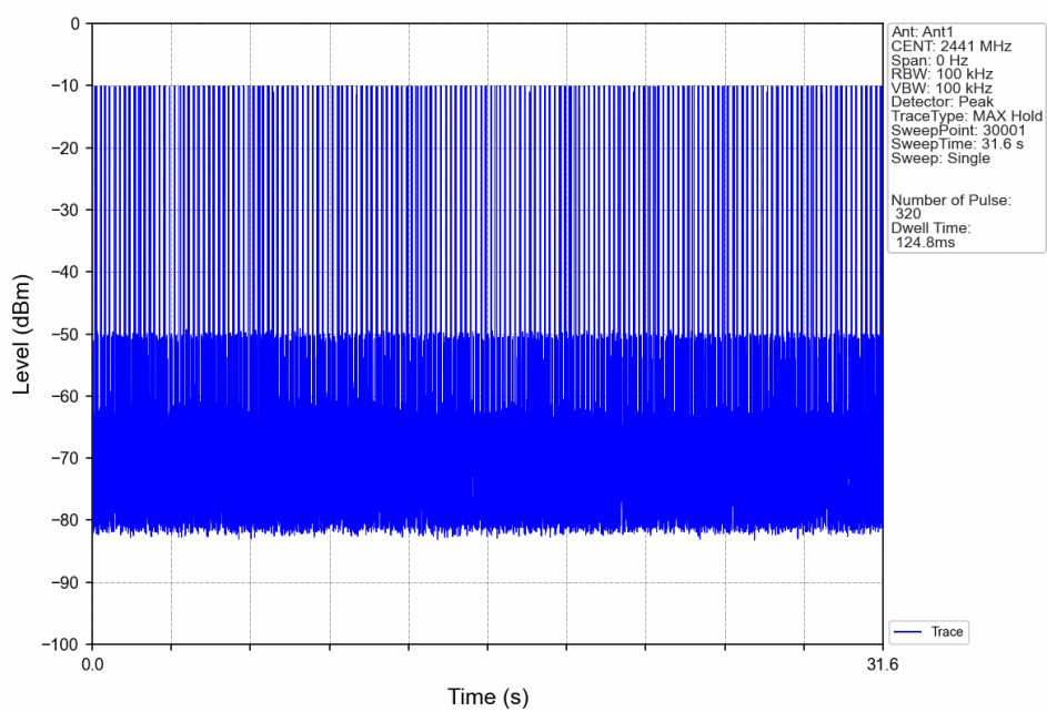
8-DPSK_3DH1_HOPP_Ant1_NTNV
