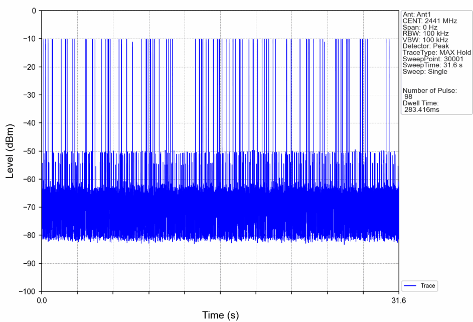
8-DPSK_3DH5_HOPP_Ant1_NTNV
