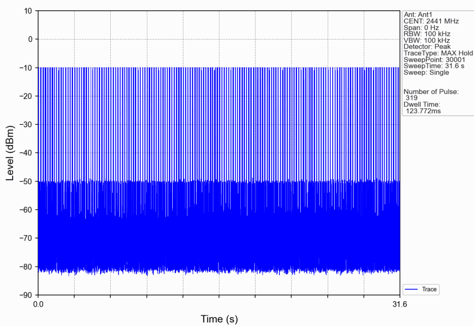
\pi/4 -DQPSK_2DH1_HOPP_Ant1_NTNV
