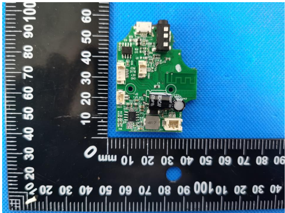
Original IC
