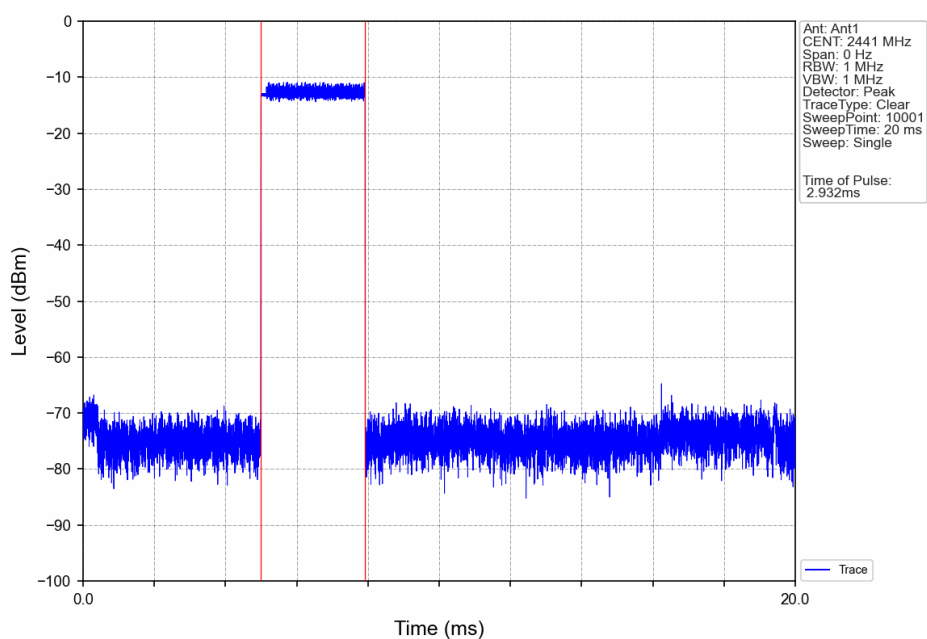
8-DPSK_3DH5_HOPP_Ant1_NTNV
