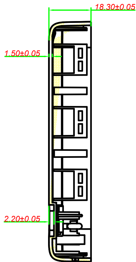
截面图
