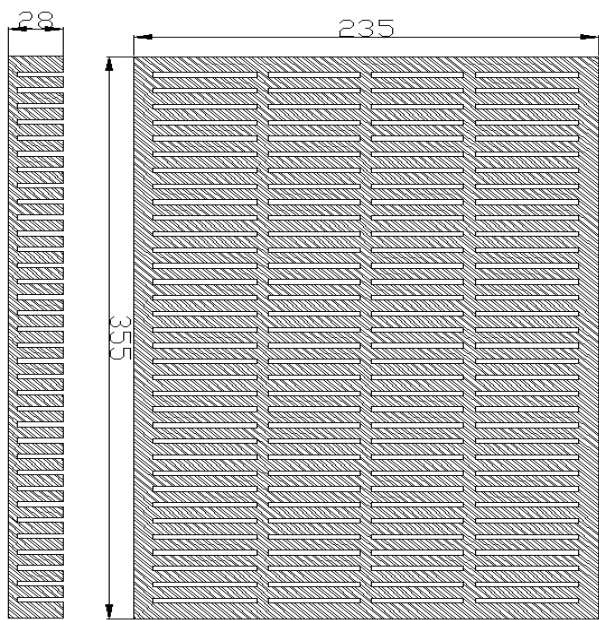
侧面图
